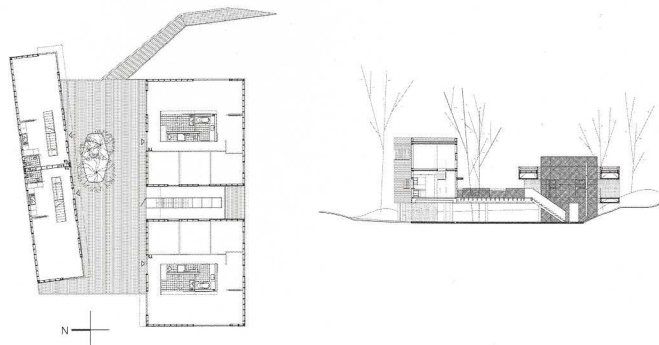
Grundriss Eingangsebene und Schnitt Floor plan entrance level and section
